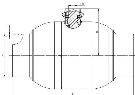
Wymiary
