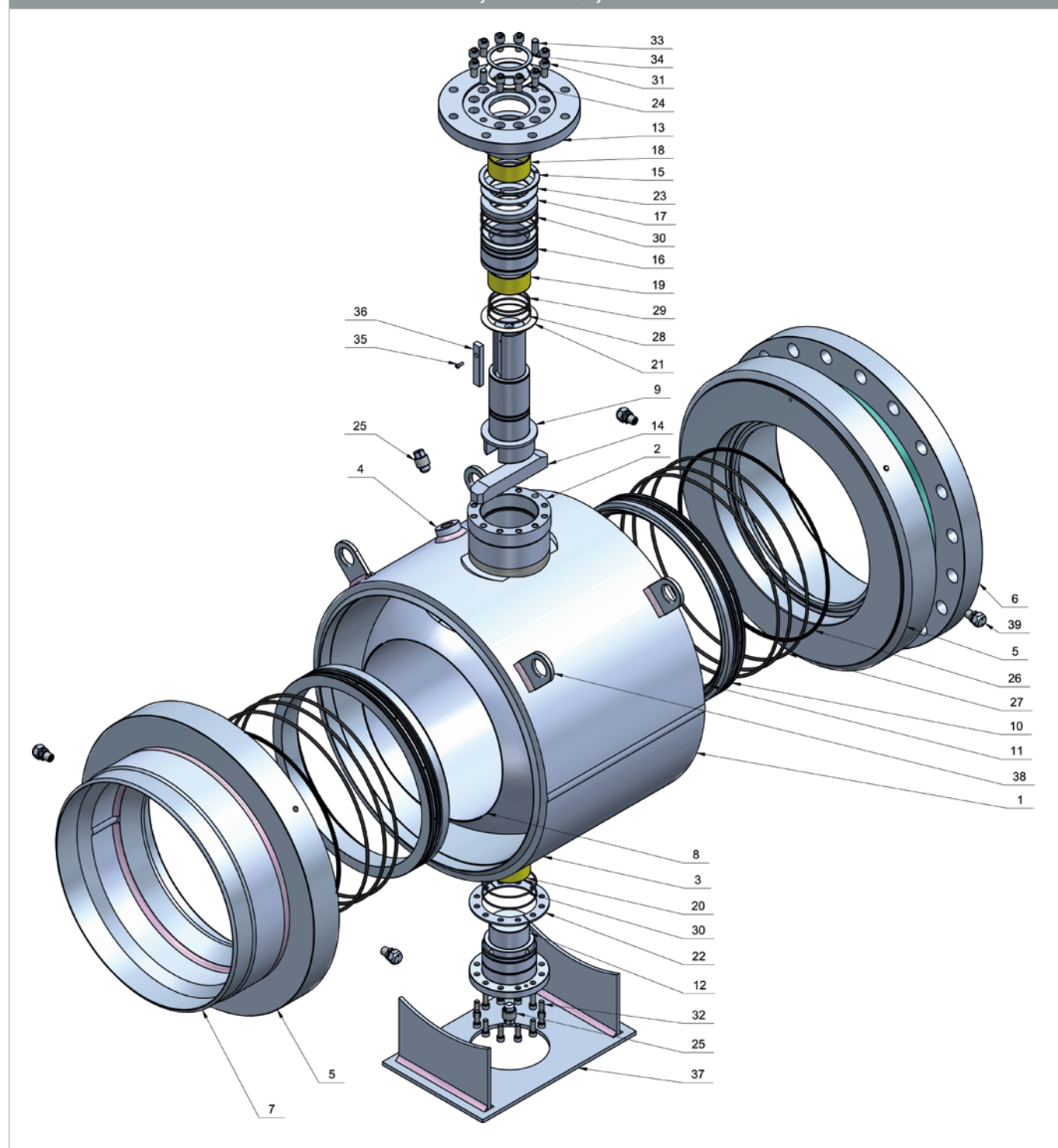
Rysunek techniczny
