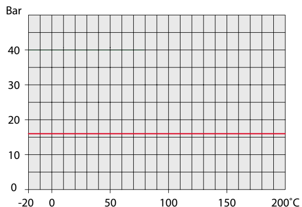
PN 16: Do wspawania x Do wspawania / Kołnierz x Kołnierz - DN 700 - 1000
